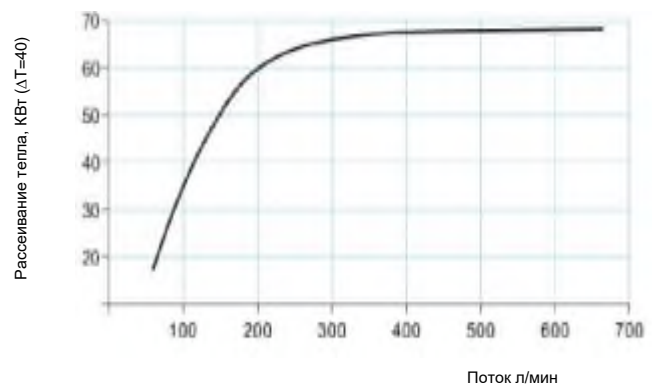
Кривые производительности
