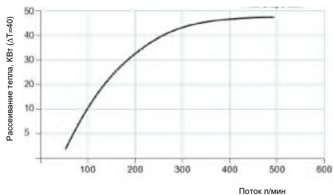
Кривые производительности
