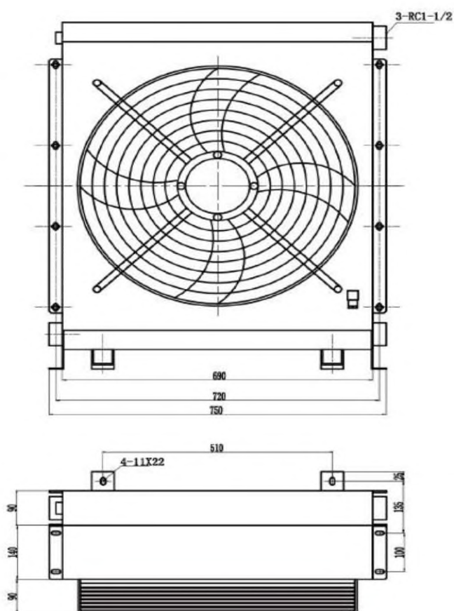
Эскизный чертёж
