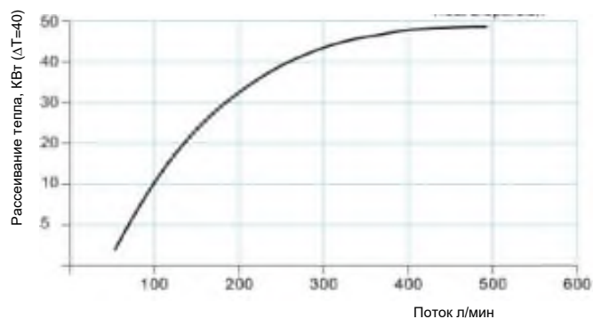
Кривые производительности
