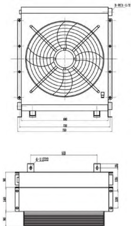
Эскизный чертеж
