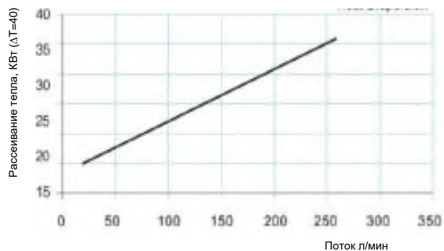
Кривые производительности
