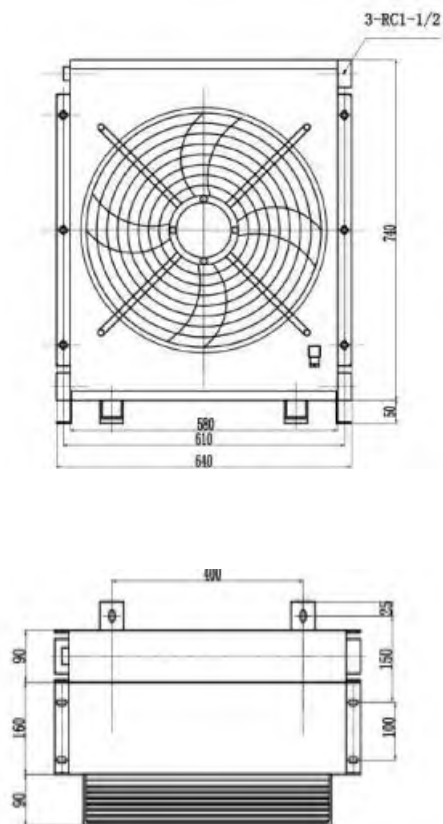
Эскизный чертёж
