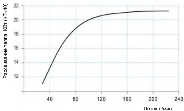
Кривые производительности
