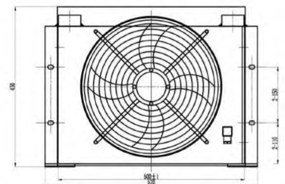
Эскизный чертёж
