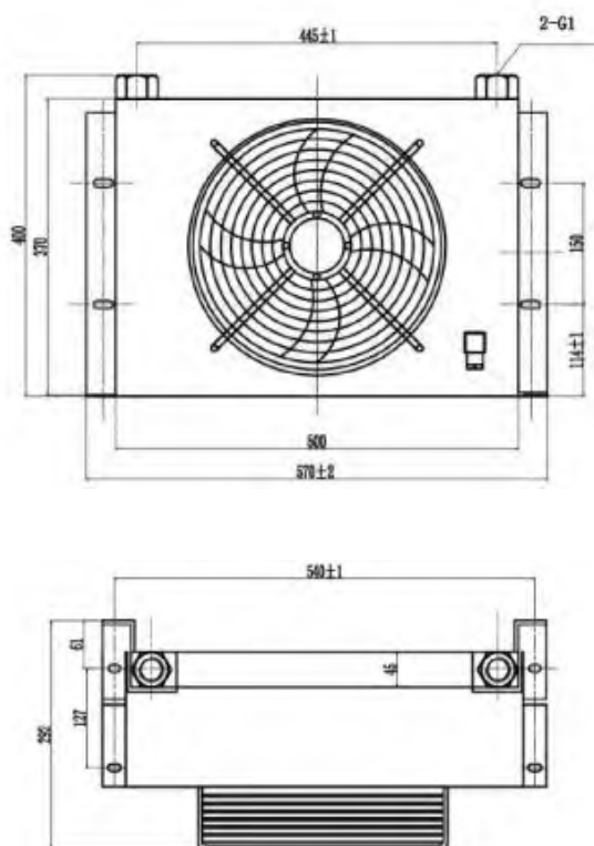
Эскизный чертёж
