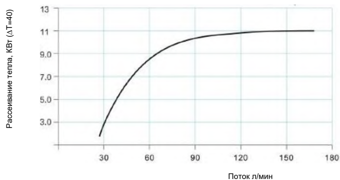
Кривые производительности
