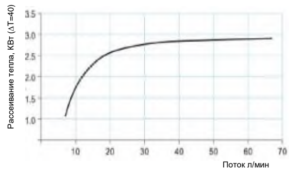
Кривые производительности
