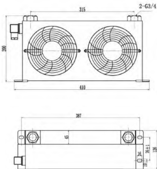
Эскизный чертёж
