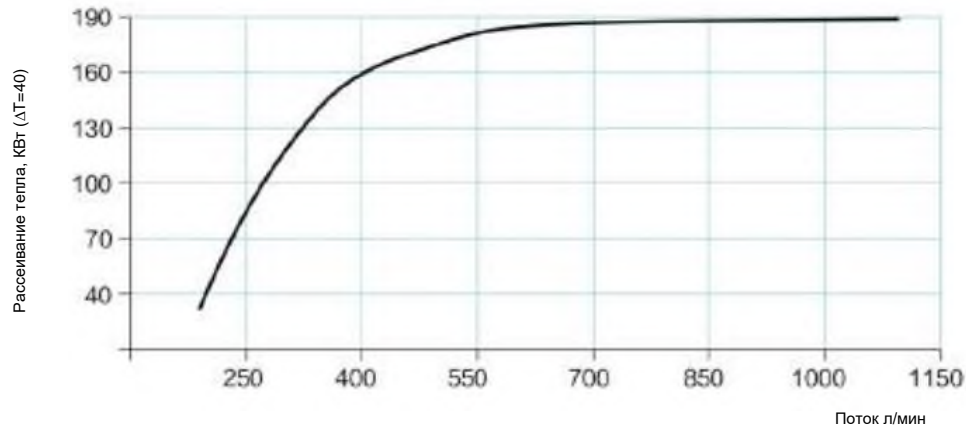
Кривые производительности
