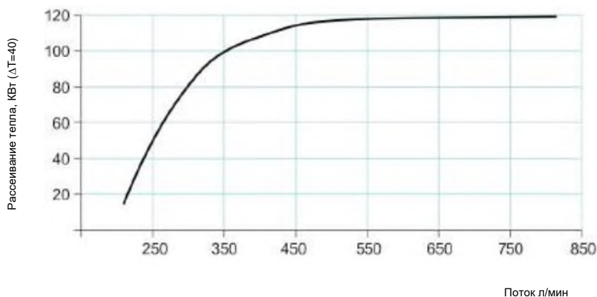
Кривые производительности
